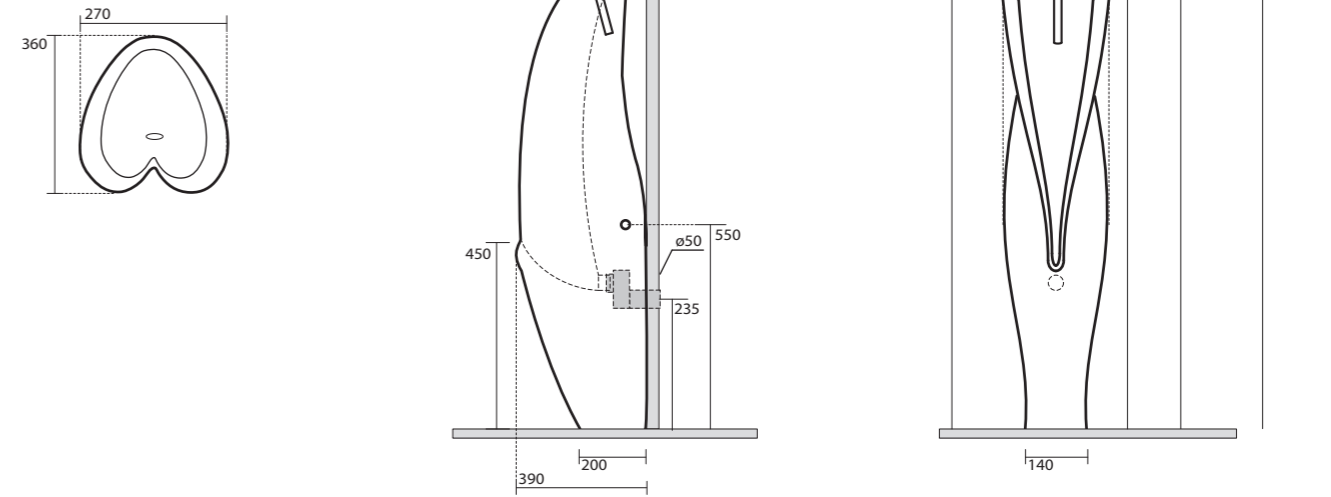
7565 Dispositivo di cacciata a parete per orinatoi Concealed urinal flush valve
